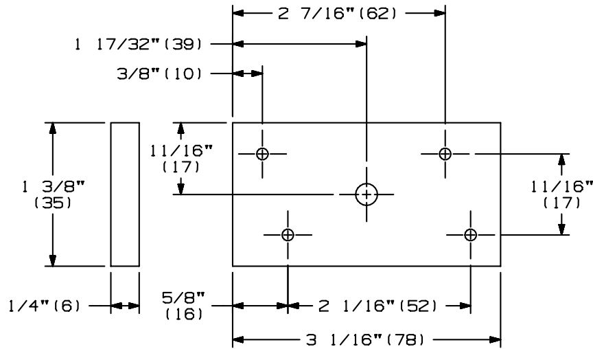
JAMB BRACKET
